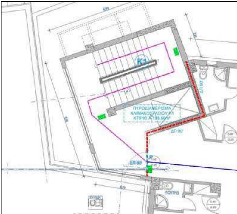
Κάτοψη 2 ου ορόφου
